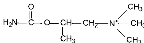
Betanechol
