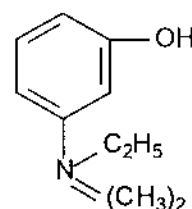
Tensilon
