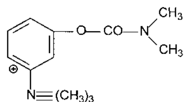
Prostigmin
