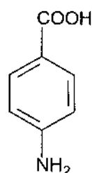
PABA
