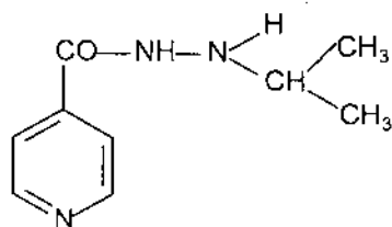
Iproniazid
