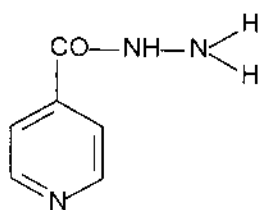
Isoniazid
